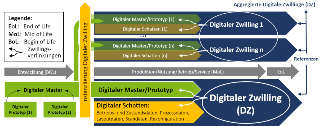
Abbildung 1: Definition des Digitalen Zwillings in Abhängigkeit von Produkt (unten) und Produktinstanz (oben) sowie Digitalem Master bzw. Prototyp und Digitalem Schatten
