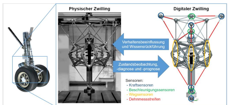
Abbildung 3: Demonstrator zur experimentellen Verhaltensanalyse eines Flugzeugfahrwerks mit Sensorik zur Anknüpfung an den digitalen Zwilling [14, 15]
